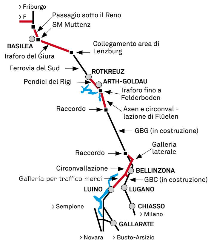
Proposta per una nuova linea per i treni merci in transito attraverso la Svizzera. In nero: sezioni di tratte esistenti o in costruzione. In rosso: nuovi elementi di tratta: galleria di base del Ceneri (GBG) e galleria di base del San Gottardo (GBC). (Grafico: Rolf Signer)
