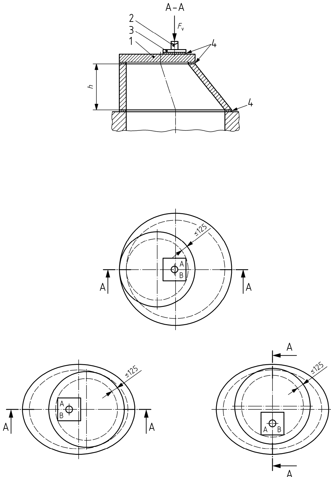
Bild B.2 — Prüfung der vertikalen Scheitelbruchlast für Konen
