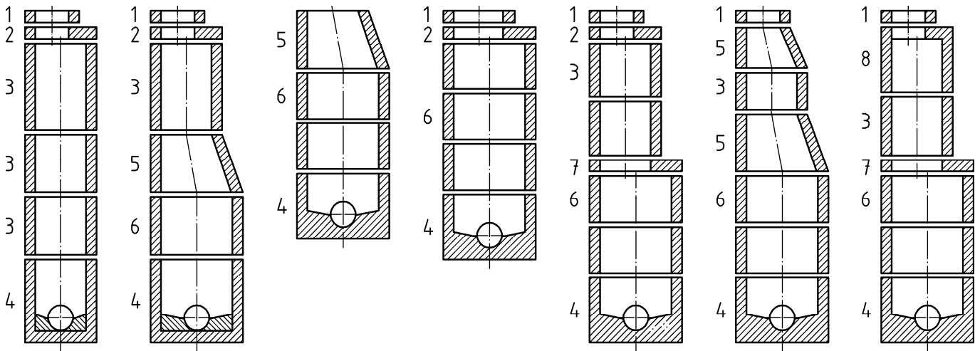
Bild 1 — Typische Bauteile
