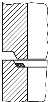
Figure 2.b) — Garniture d'étanchéité élastomère ou plastomère ou autres matériaux d'étanchéité
