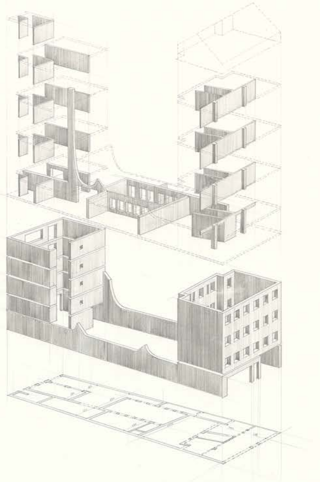
Axonometrie Tragwerk
